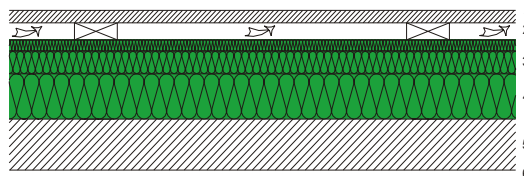
Voorbeeld 2 Isolatie achter een beluchte gevelbekleding
