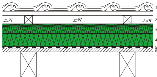
Voorbeeld 1 Isolatie over het dakbeschot onder de dakpannen
